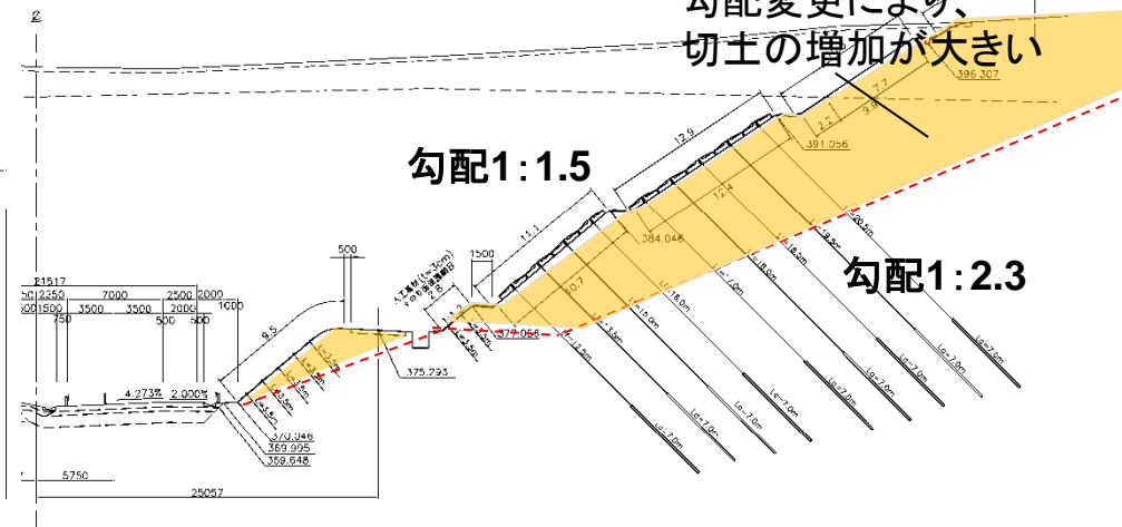
B-B'断面
