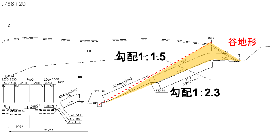
A-A'断面
