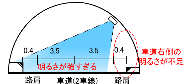
2車線トンネル (右片側配列セラメタ)
