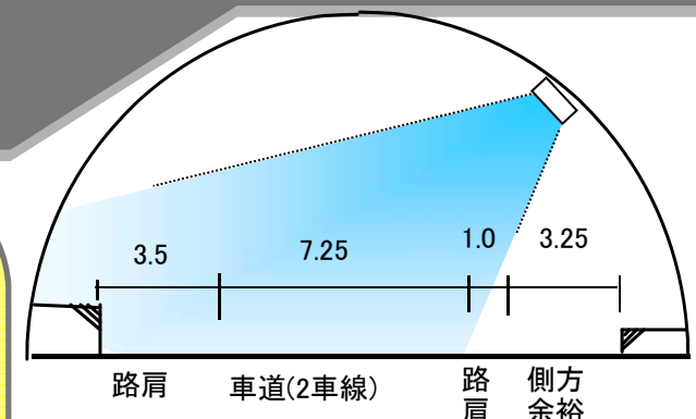
大断面トンネル (右片側配列セラメタ)
