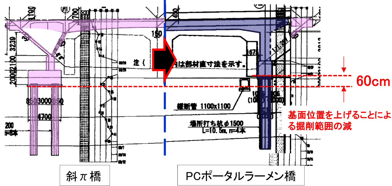
橋梁形式の変更
