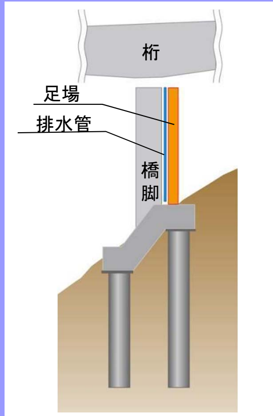
一般構造物用足場を設置した例
